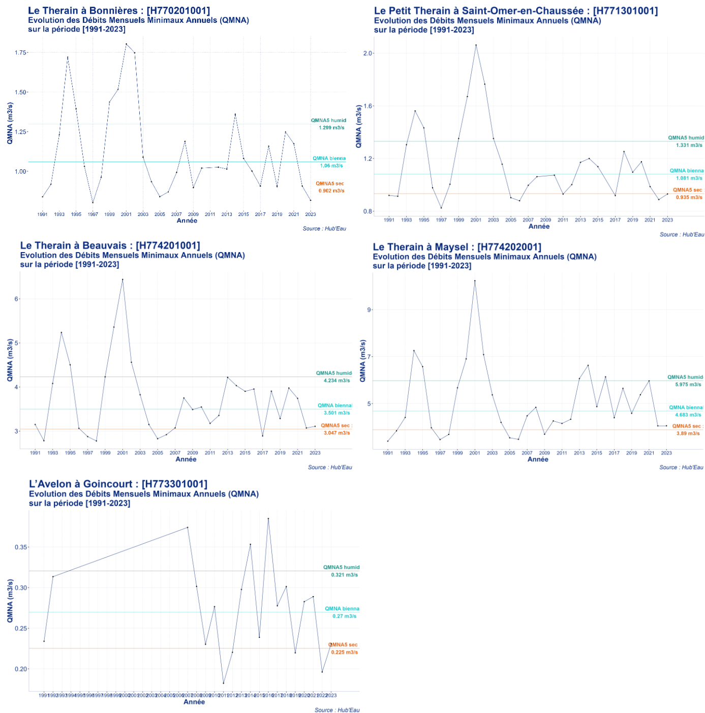
Figure 14 : Evolution des QMNA aux différentes stations vis-à-vis du QMNA quinquennal (sec et humide) et du QMNA biennal
