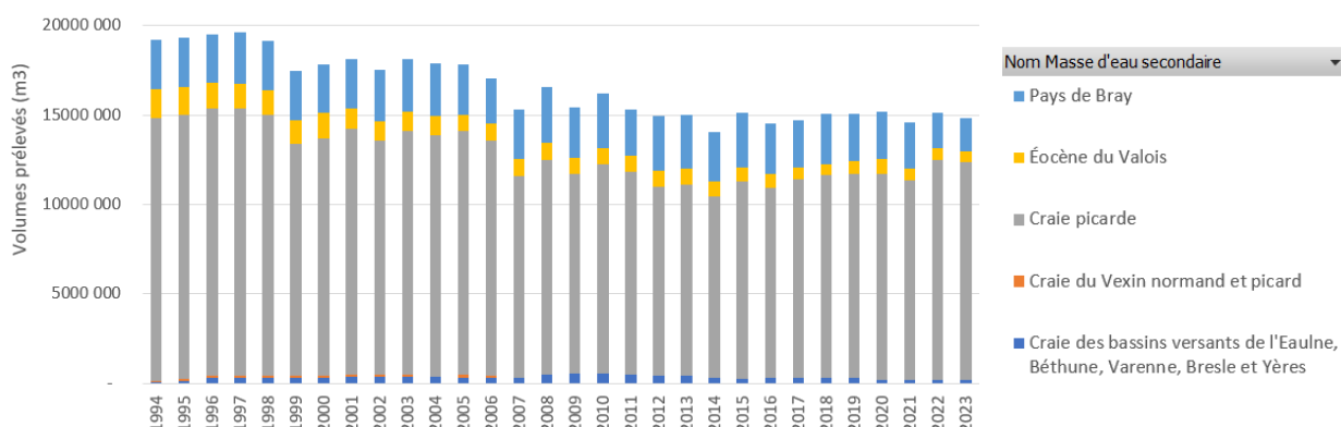
Figure 32 : Evolution des prélèvements annuels en eaux souterraines selon les masses d'eau captées
