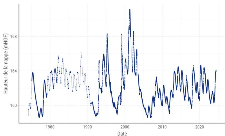
Figure 8 : Chronique journalière d'un piézomètre amont sur la nappe de la Craie, à double cyclicité annuelle : BSS000FNLM à Omecourt
