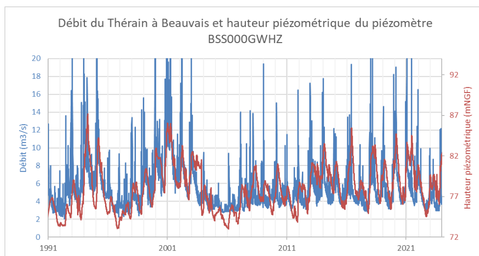
Figure 12 : Comparaison entre le débit du Thérain à Beauvais et les variations de hauteur d'eau sur le piézomètre BSS000GWHZ
