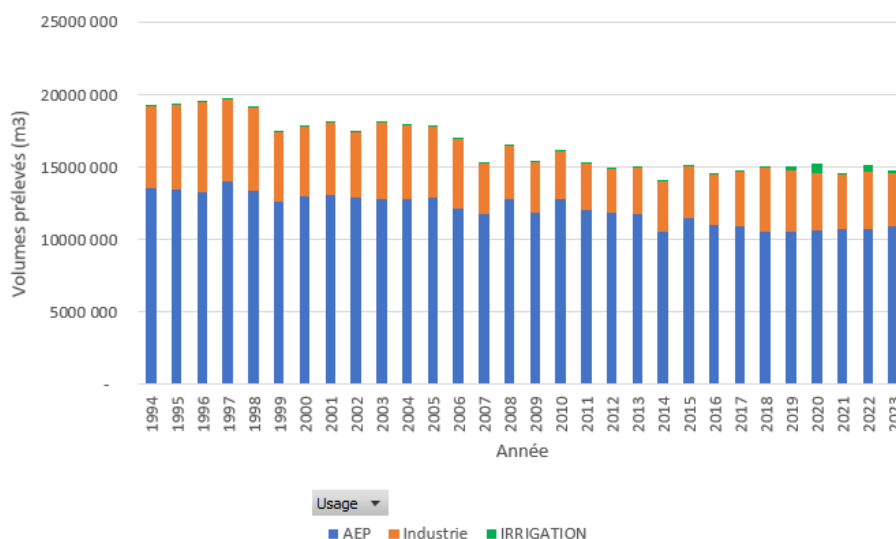
Figure 31 : Evolution des prélèvements annuels en eaux souterraines
