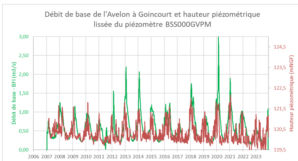
Figure 13 : Comparaison entre le débit de base de l'Avelon à Goincourt (calculé par la méthode de Wallingford) et les variations de hauteur d'eau sur le piézomètre BSS000GVPM (moyenne glissante sur 9 jours)
