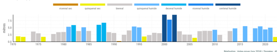
Figure 24 : Recharge, vidange et solde apparents en mètres de niveau d'eau dans le piézomètre BSS000GXKH à la Craie Picarde, et période de retour associée
