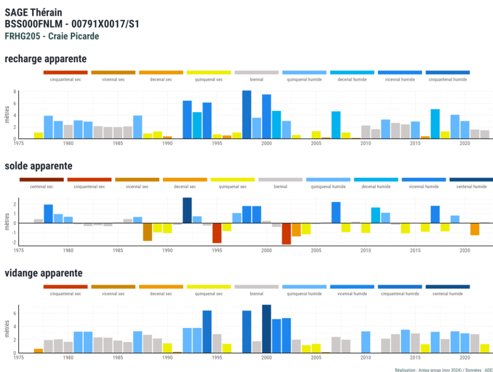
Figure 23 : Recharge, vidange et solde apparents en mètres de niveau d'eau dans le piézomètre BSS000FNLM à la Craie Picarde, et période de retour associée
